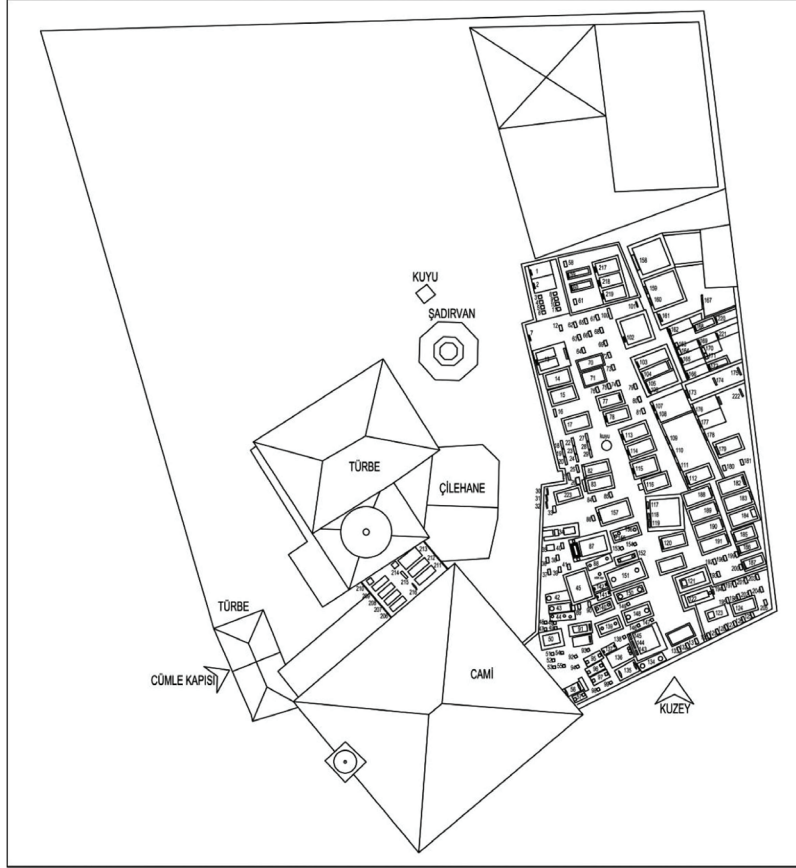
Plan I: Merkez Efendi Külliyesi Genel Planı.
